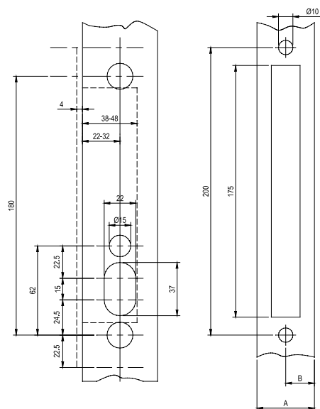
5049 - aluminium door
