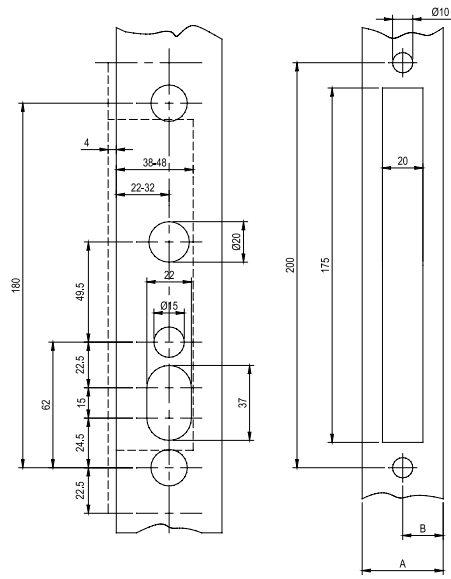
5016 - aluminium door
