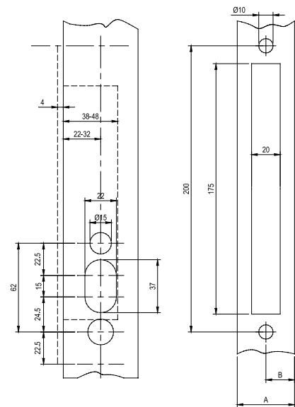
5018/5032 - aluminium door
